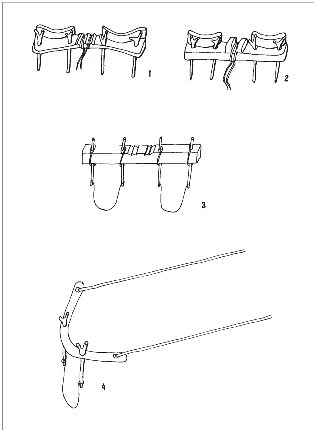
Tafel IX: Jochtypen 1-3 Doppeljoch 4 Einzeljoch
