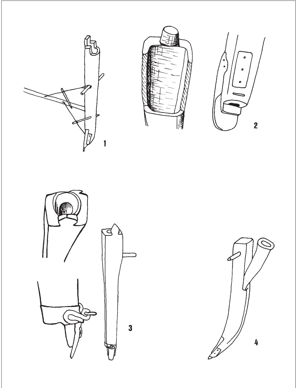
Tafel VIII: 1 Sohlenlose Arl 2 links: Einwurföffnung für das Saatgut 2 rechts: Ausgangsöffnung des Saatgutes mit der Pflugschar 3 eine Variante von 2 4 Sohlenlose Arl mit eingesetztem Ledersack, vgl. Tafel V.1 rechts
