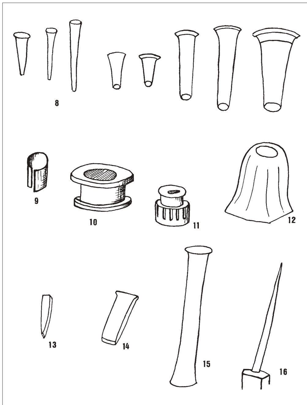
Tafel XXVIII: Schmiedewerkzeuge 8 Warmschrotmeißel 9–12 Rundgesenke 13–15 Kaltschrotmeißel 16 Stichel
