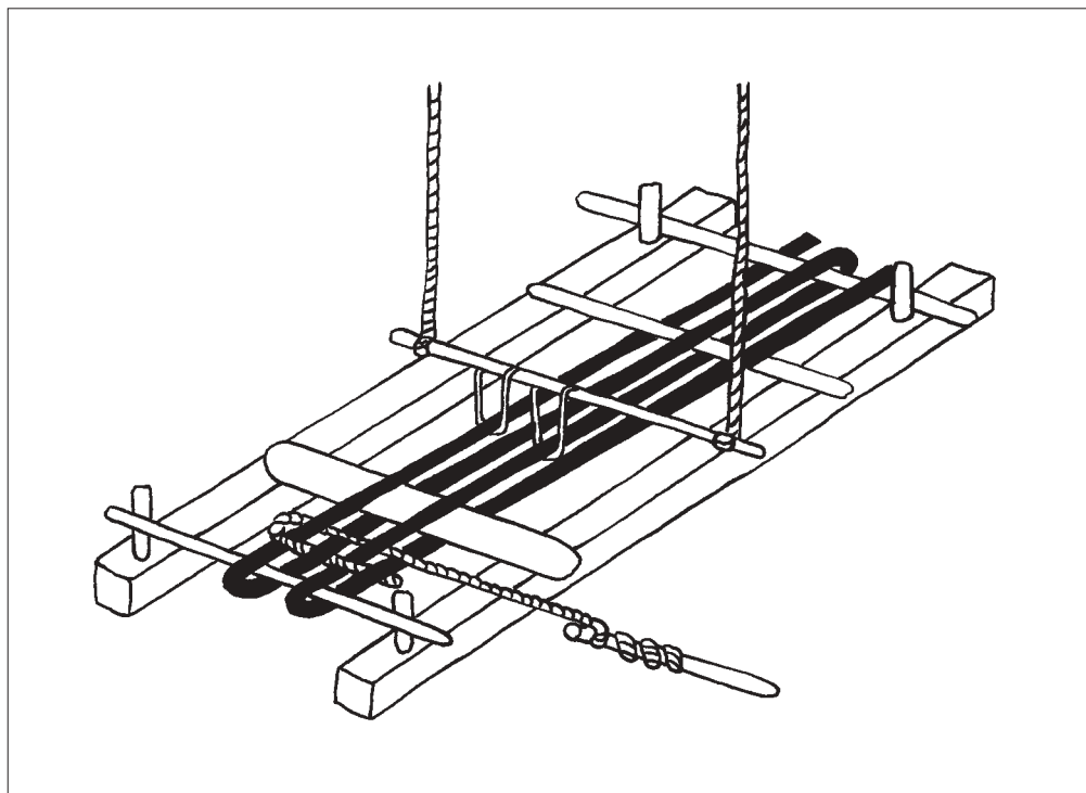
Tafel XX: Horizontales Webgerät
