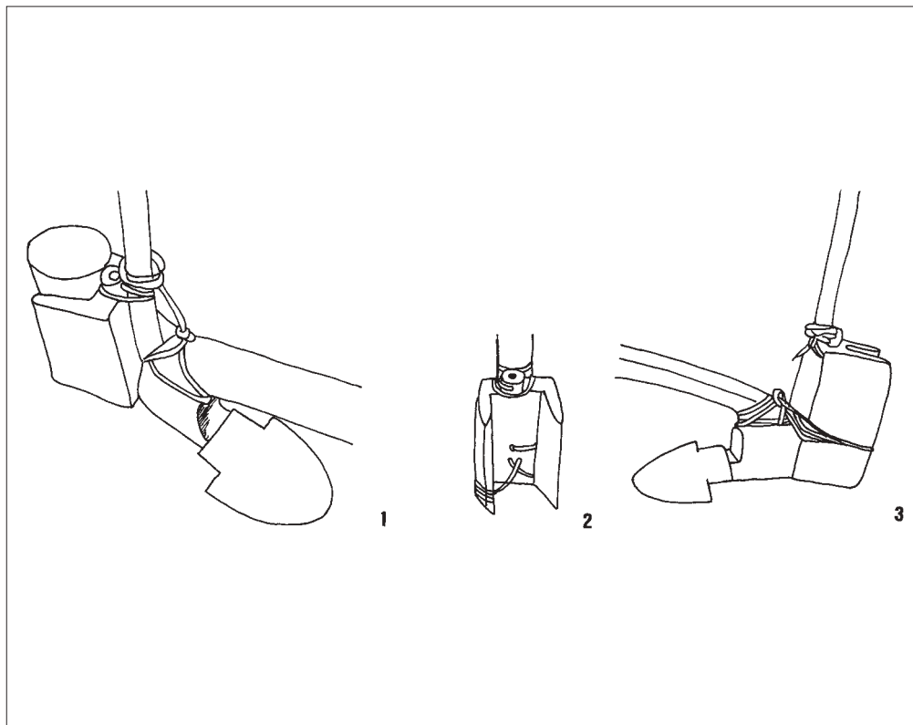
VII: 1-3 Kastenartige Behälter für Sättrichter
