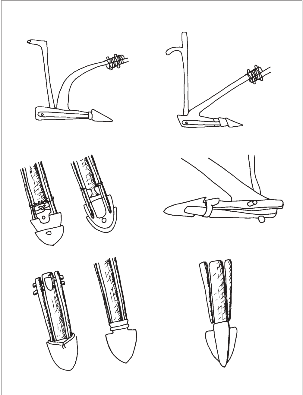
Tafel IV: Streichvorrichtungen
