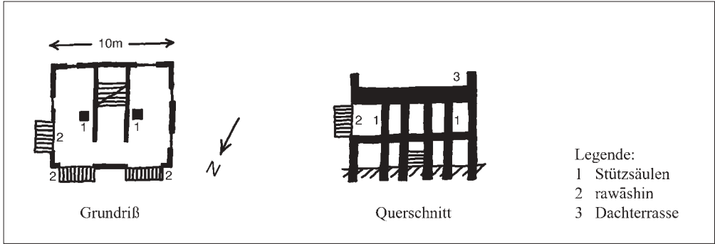
Tafel XXXIII: Einfaches Wohnhaus aus Korallenstein in al-Qunfudha
