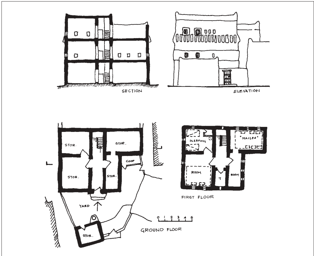
Tafel XLIII: Zwischenschacht-Gebäude des ‘Asīr
