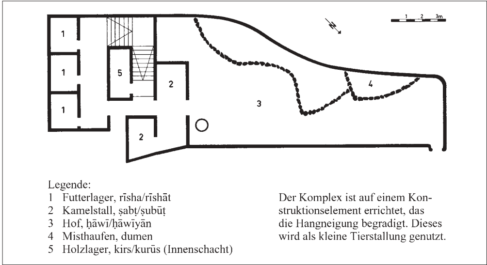
Tafel XLII: Innenschachthaus des ‘Asīr (nach: Dostal 1983c: 29)
