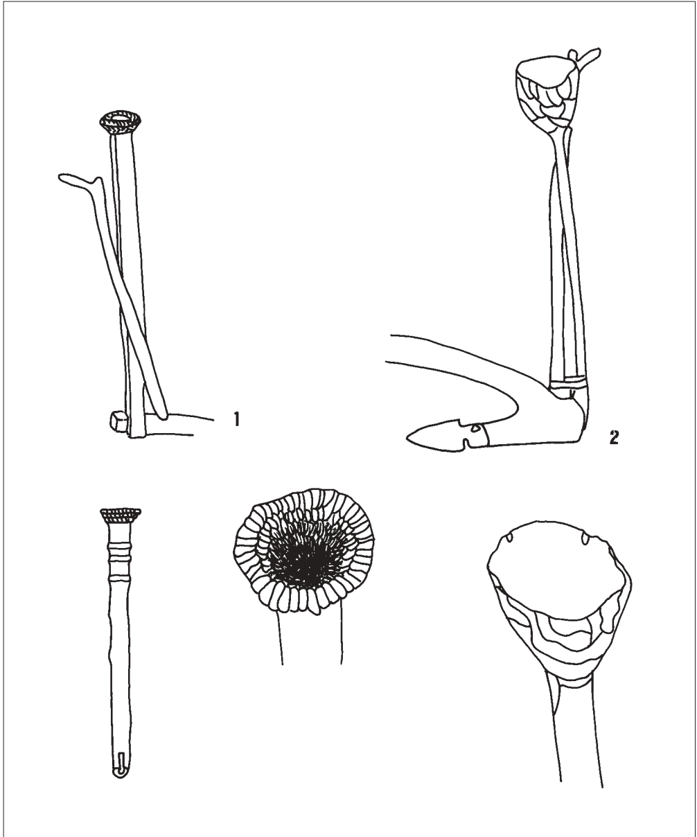
Tafel VI: 1 Sättrichter, an der Sterz angebunden 2 Sättrichter, in eine Streichvorrichtung eingesetzt unten: verschiedene Sättrichter
