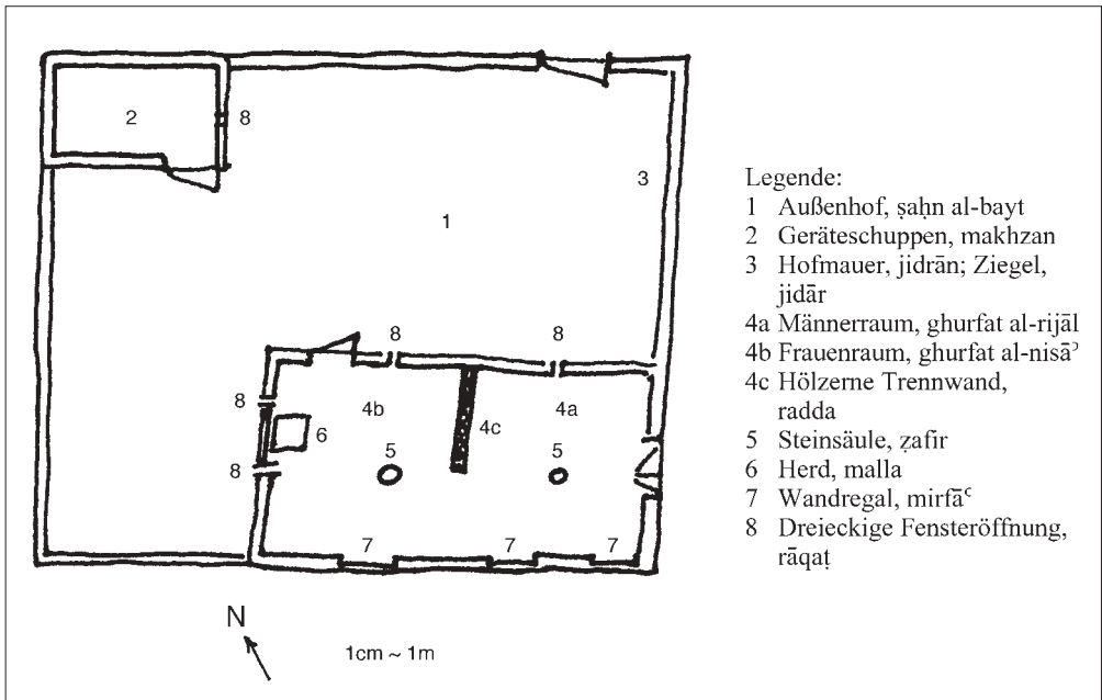
Tafel XXXIX: Lehmziegelhaus aus al-ʿAqīq im Najd-Stil (Gebäude auf Abb. 56)
