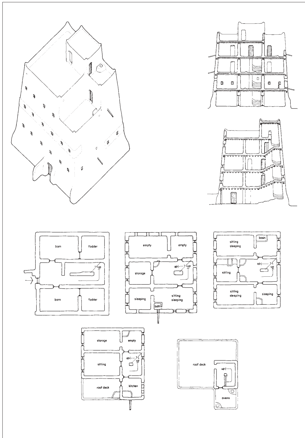
Tafel XLI: Stiegenhaus rund um eine einfache Stützmauer im 'Asir
