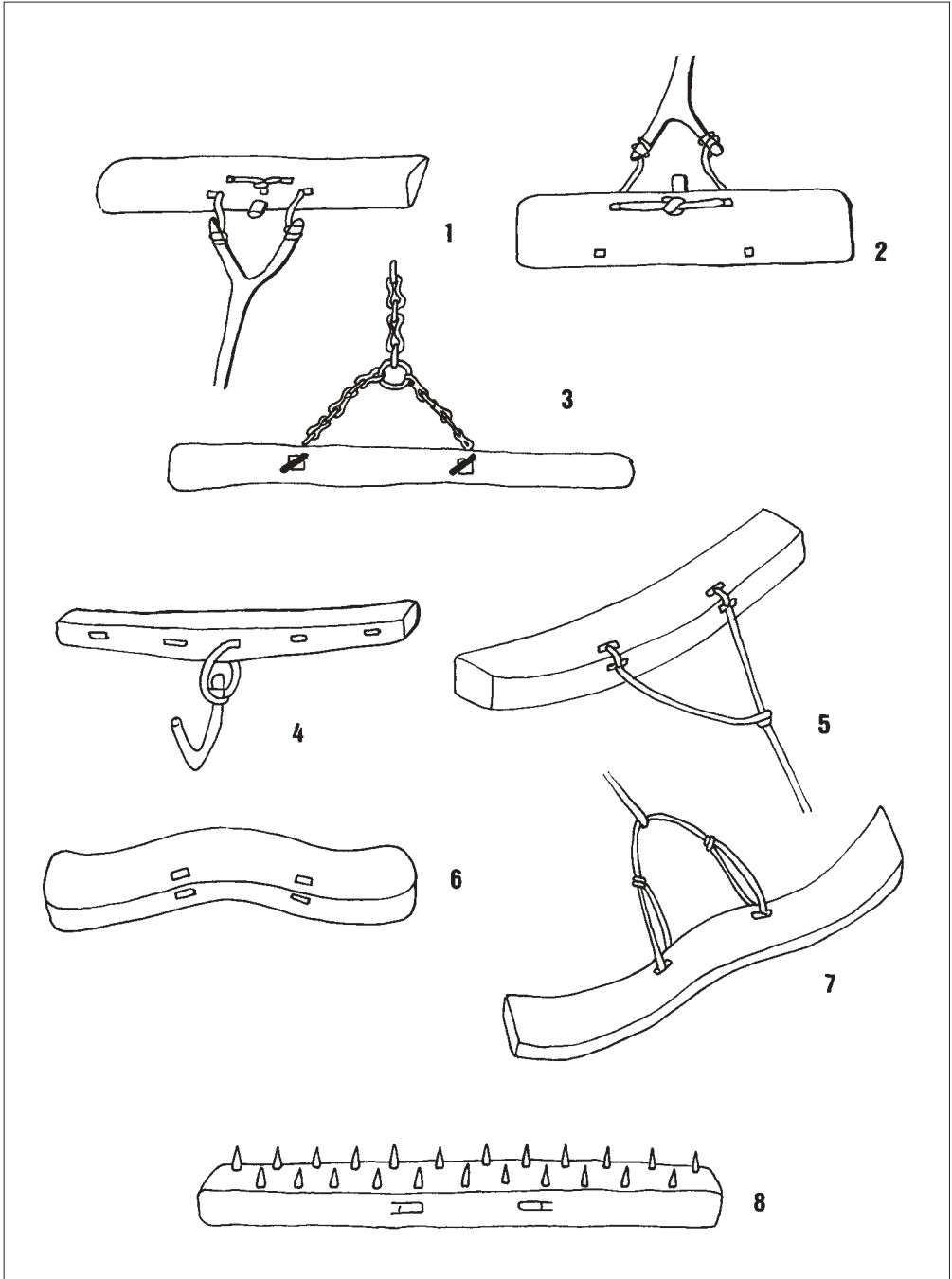
Tafel XII: 1-7 Ackerschleppen 8 Egge
