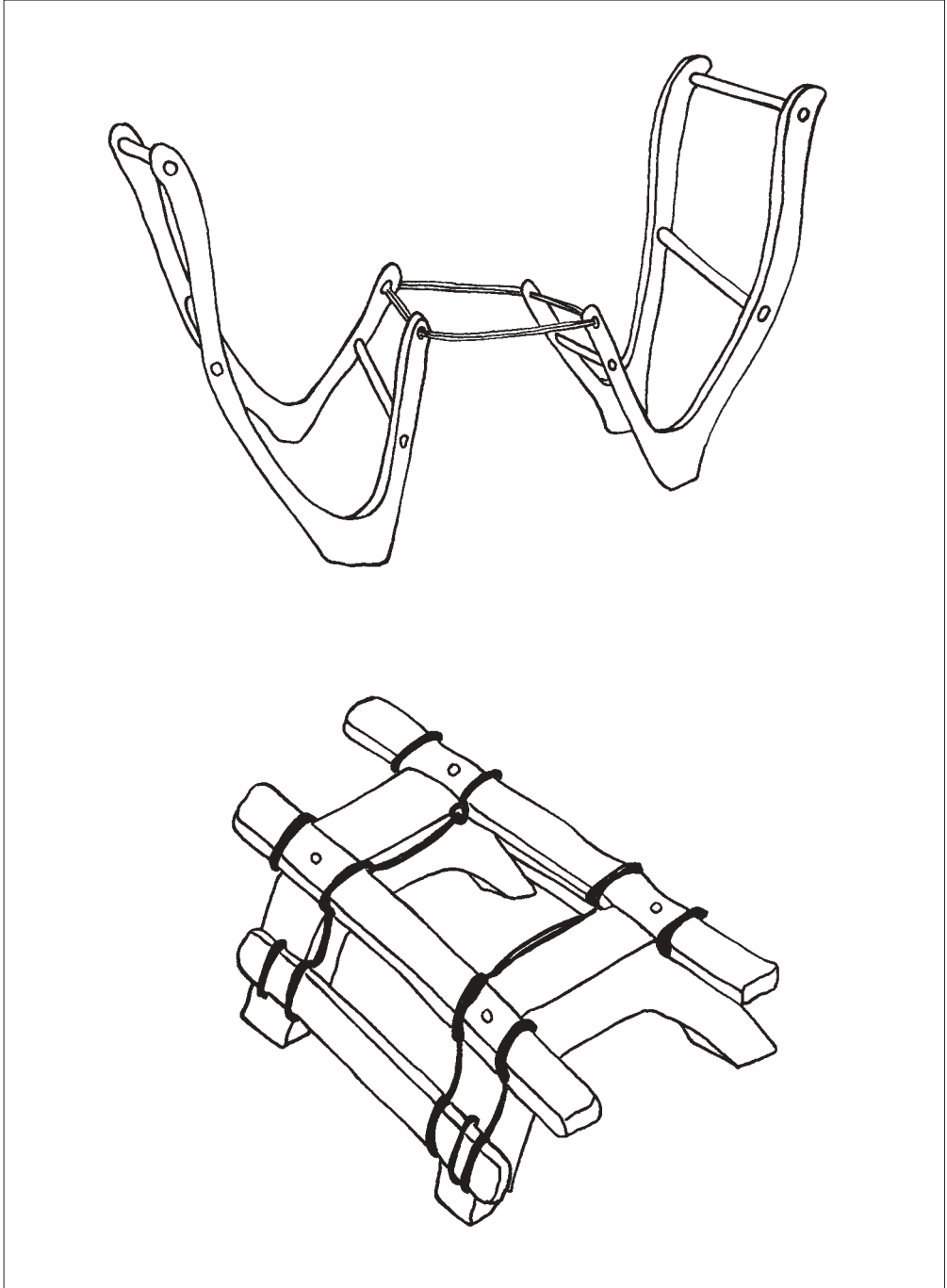
Tafel XXI: Tragsättel
