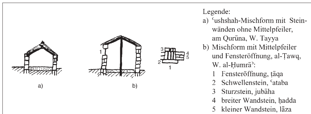
Tafel XXXVI: Mischformen am Ostrand der Tihāma
