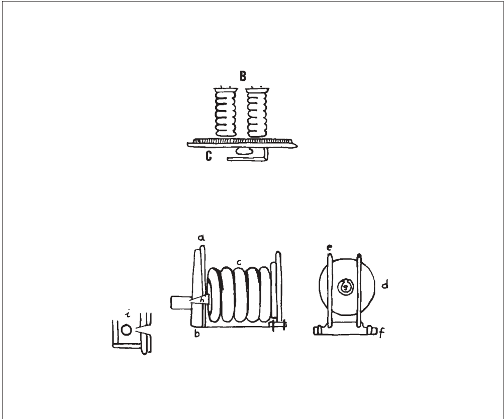
Tafel XXV: Ringgebläse
