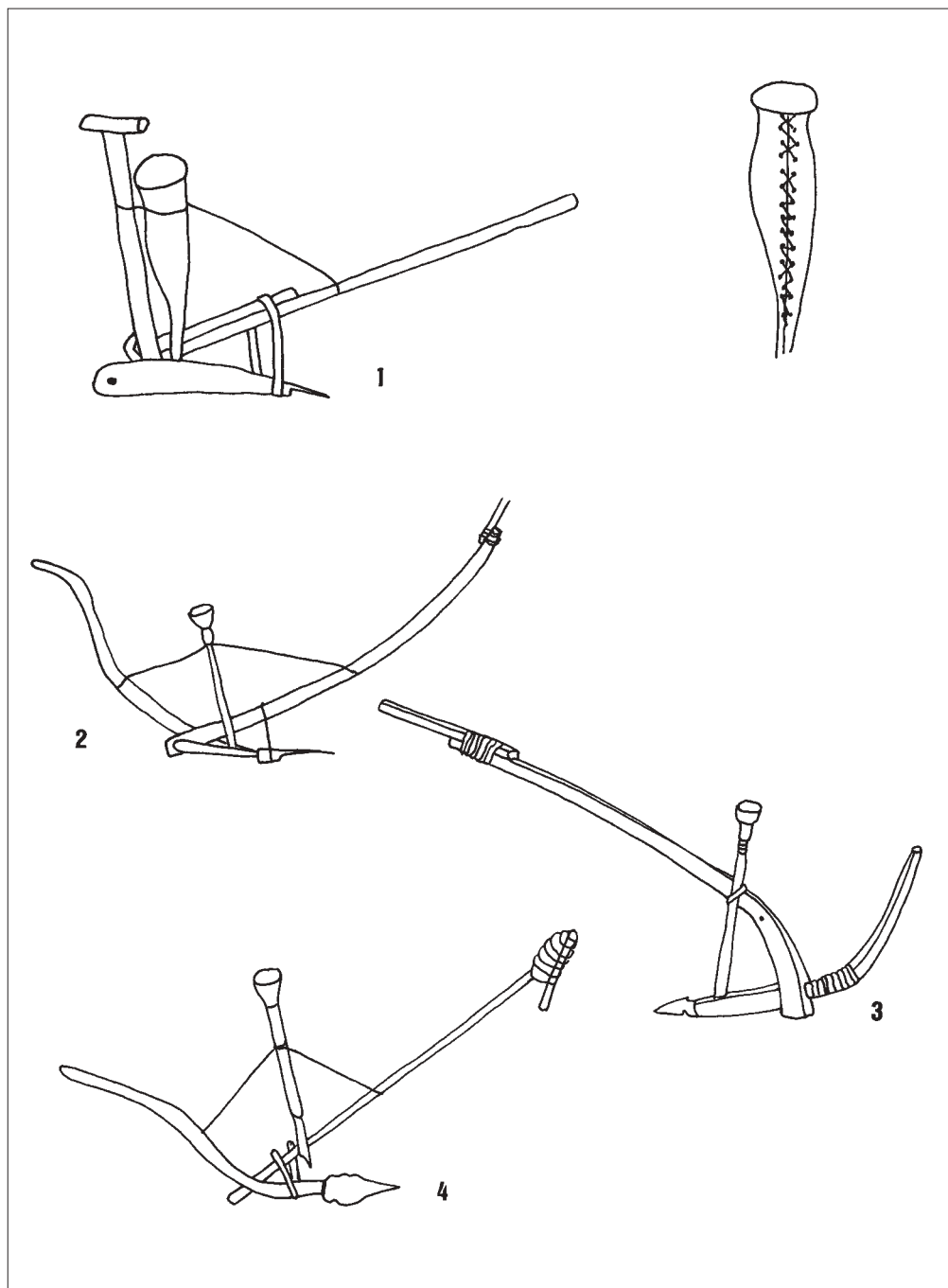
Tafel V: 1-4 Arl mit Sävorrichtung
