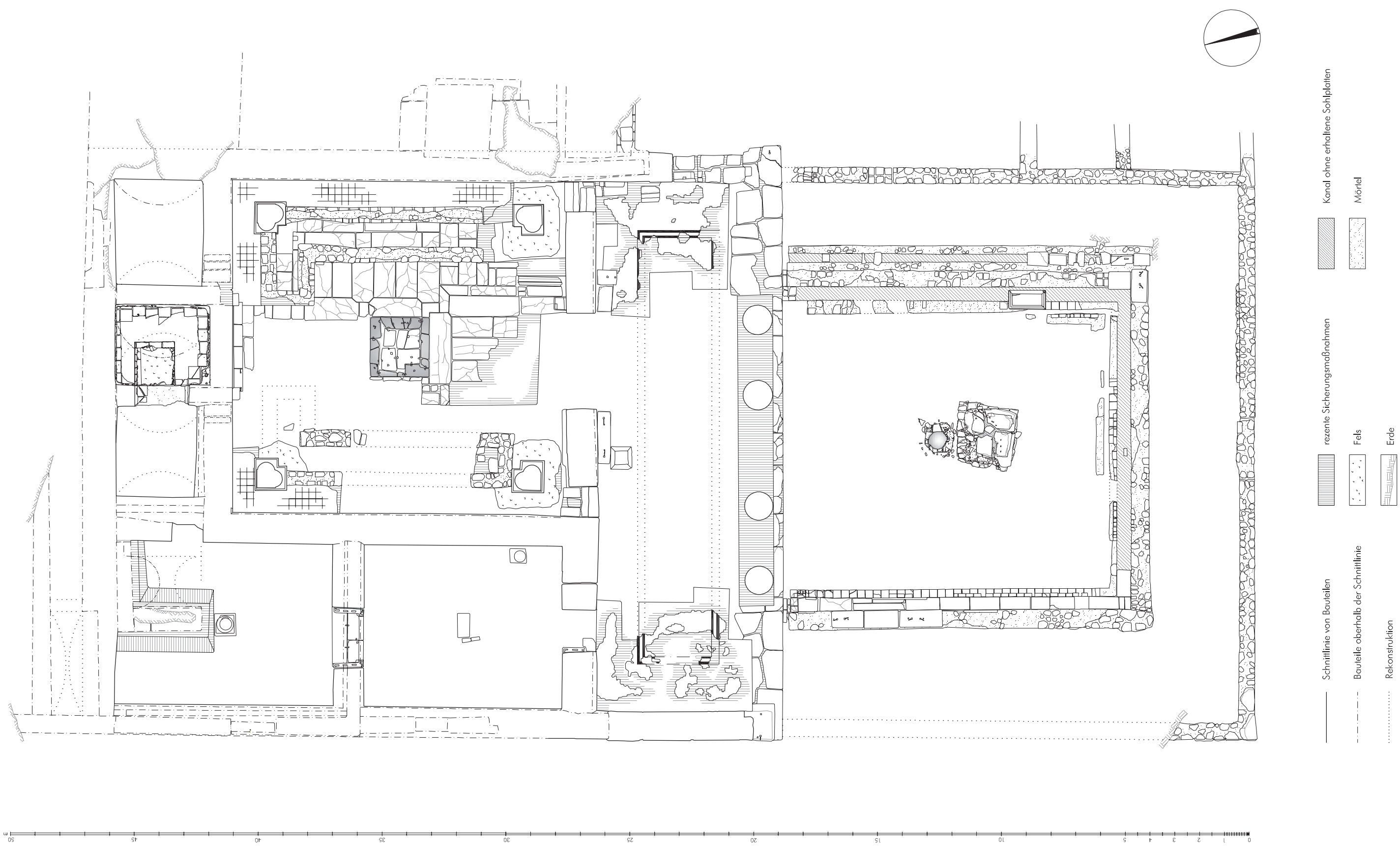
1 Prytaneion. Grundriss Bauaufnahme (1:150)
